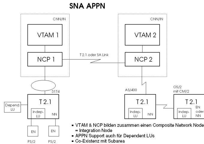
Abb. 47. VTAM/NCP als APPN Knoten
