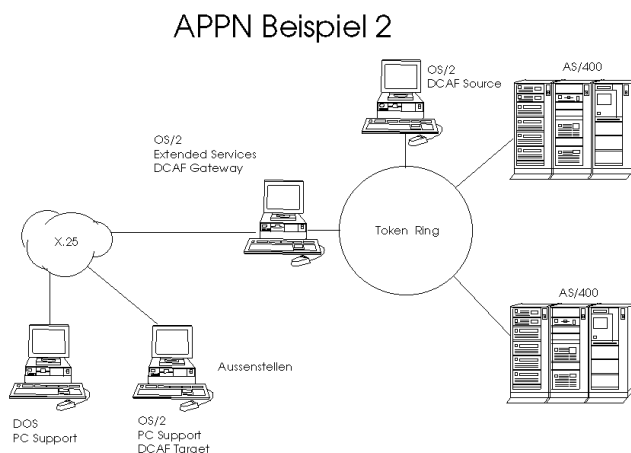
Abb. 53. APPN Beispiel mit OS/2 und AS/400
